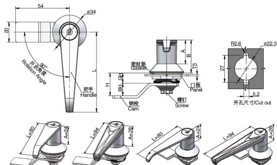
301, 301-N手柄长度图
