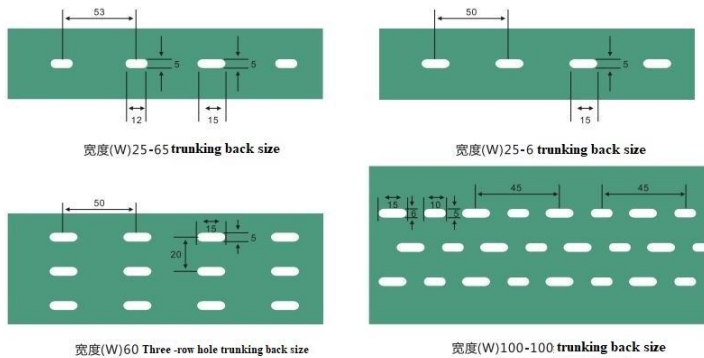
安装尺寸 ( mm ) Installation size ( mm )
